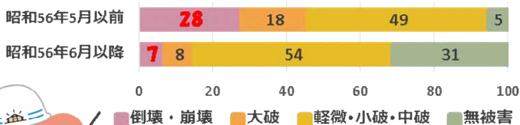
熊本地震における木造住宅被害割合 (%)
